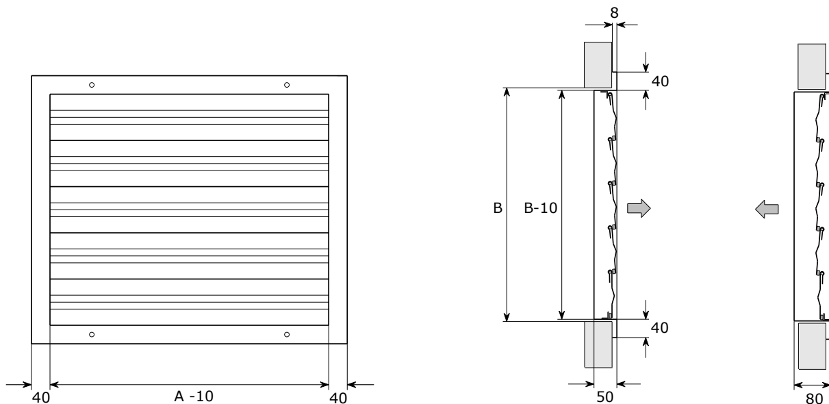
odvod / exhaust
